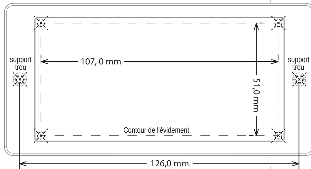
Figure 1 Modèle (échelle 1: 1)
