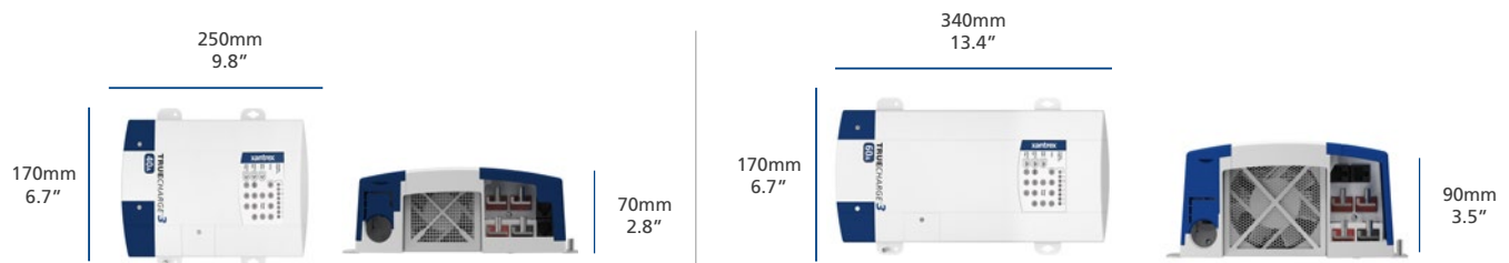
TRUECHARGE3 12V 20A &amp; 40A
